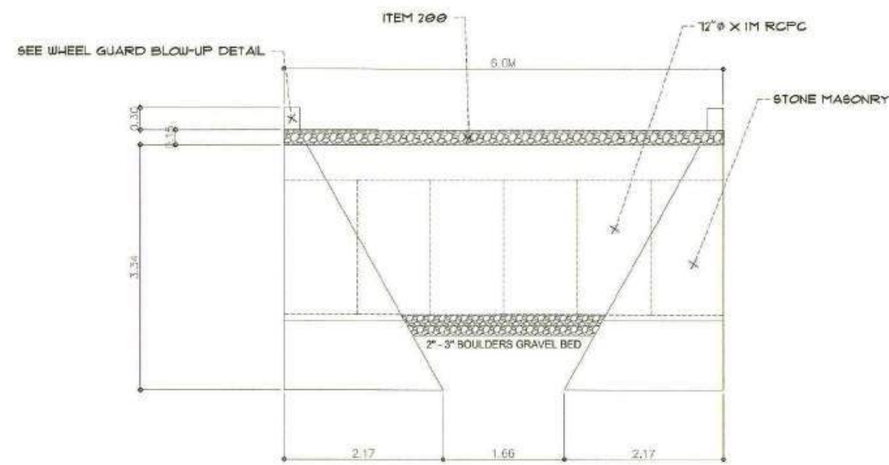
SECTION THRU-B SCALE: 1:50 M.
